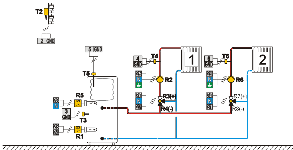
Схема 423d (WDC20) — Схема расширения — бак-теплоаккумулятор с встроеным бойлером ГВС, 2 смесительных контура
