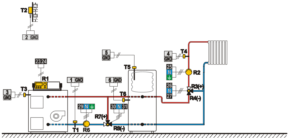
Схема 415 (WDC20) — Комбинированный котел (ТТ/ЖТ), бак-теплоаккумулятор с встроенным бойлером ГВС, смесительный контур
