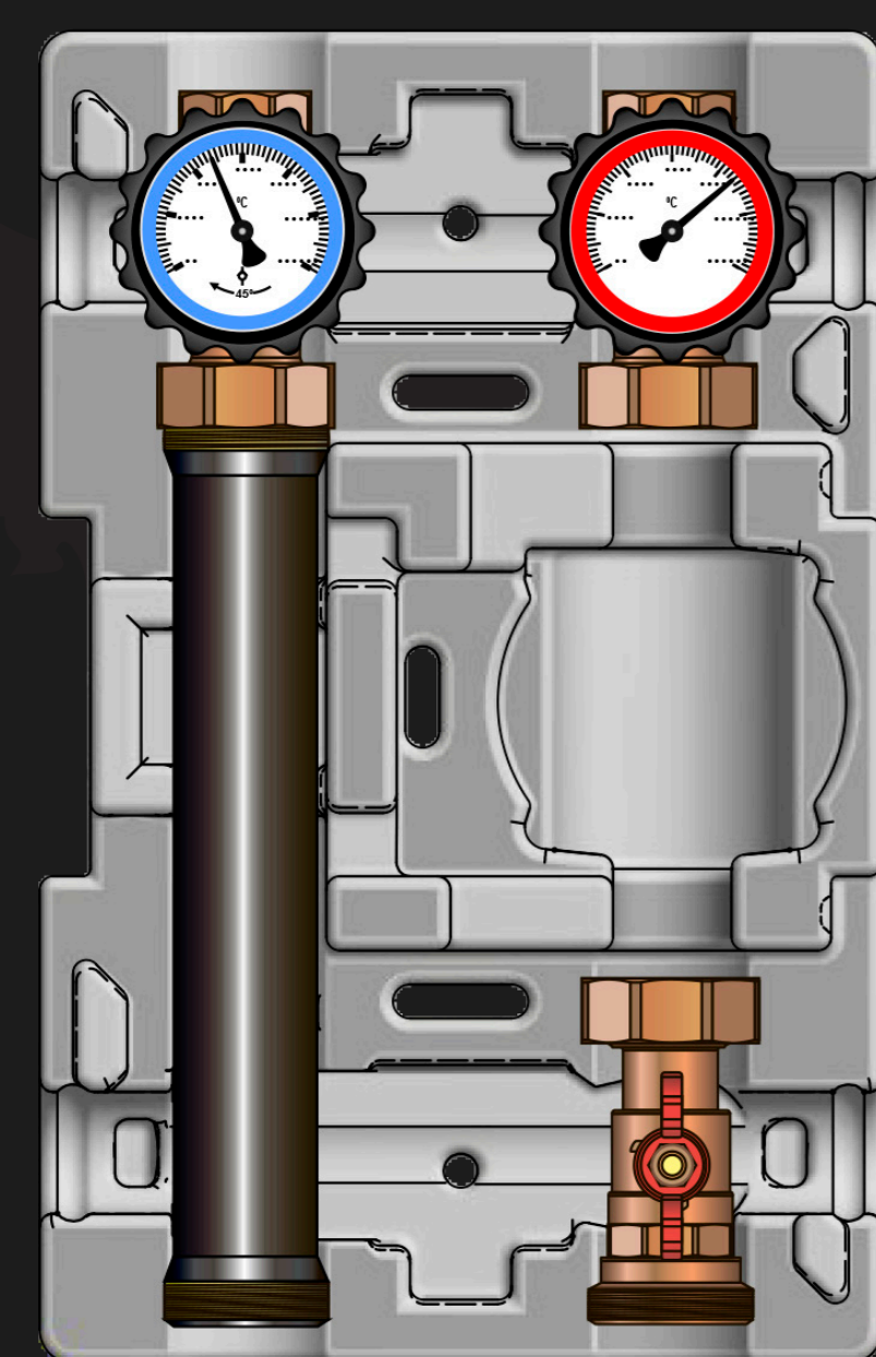
Прямую насосную группу DN25 (арт. 101.30.025.00, без насоса)
