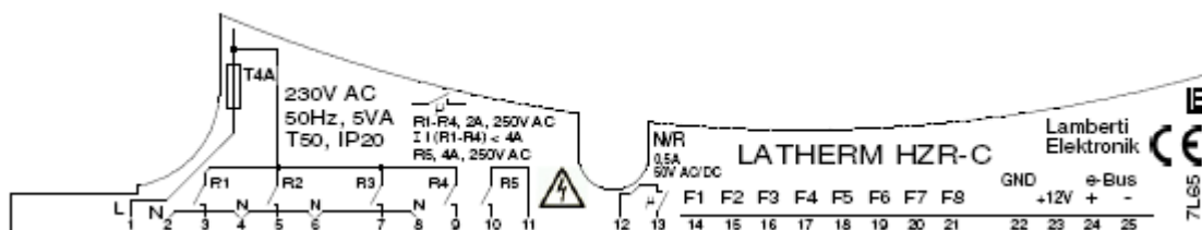
Схема подключения устройства HZR-C
